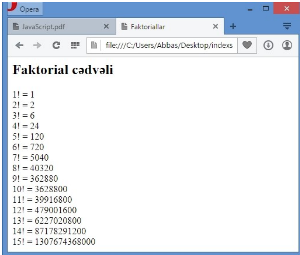
Şəkil 1.2. JavaScript-də faktorial siyahısı alqoritmi
